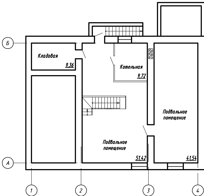
План подвала
