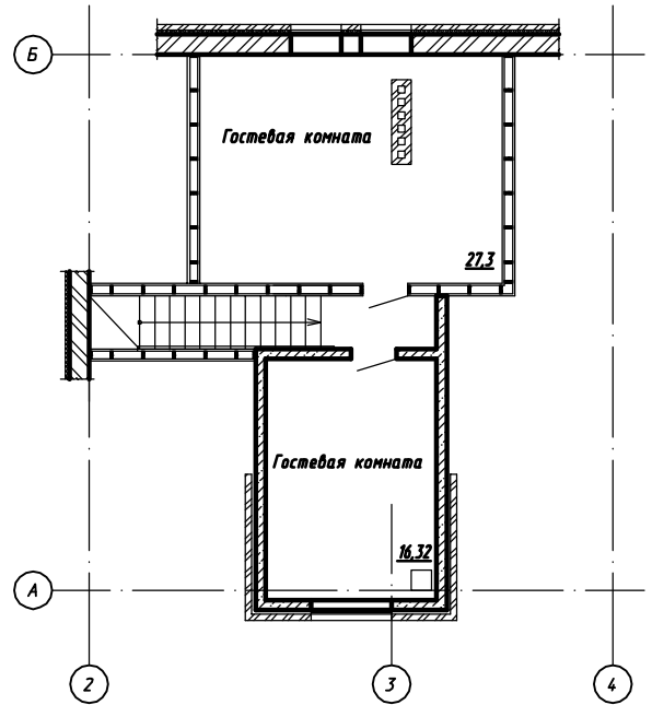
План мансарды
