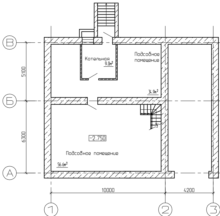
План подвала
