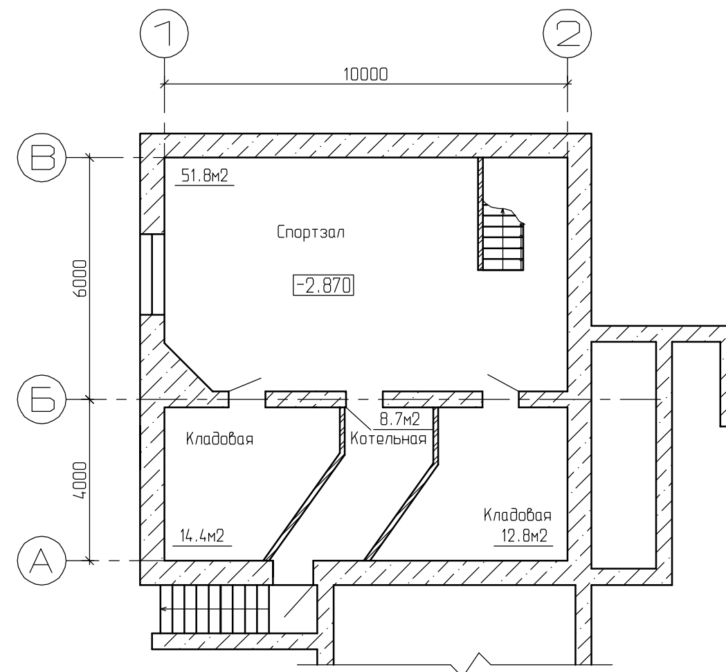
План подвала
