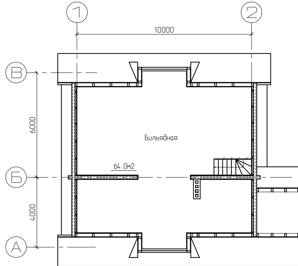
План мансарды
