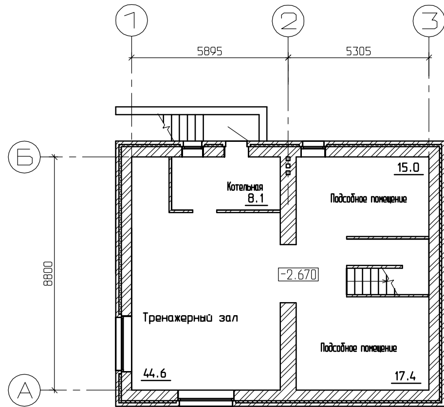
План подвала
