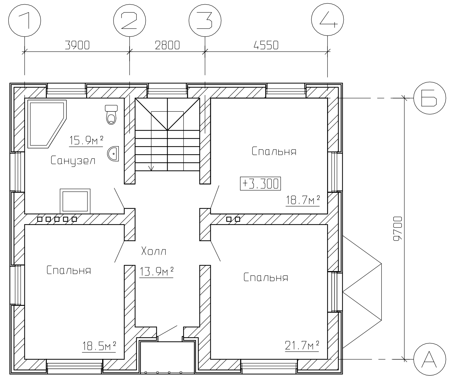
План 2-го этажа
