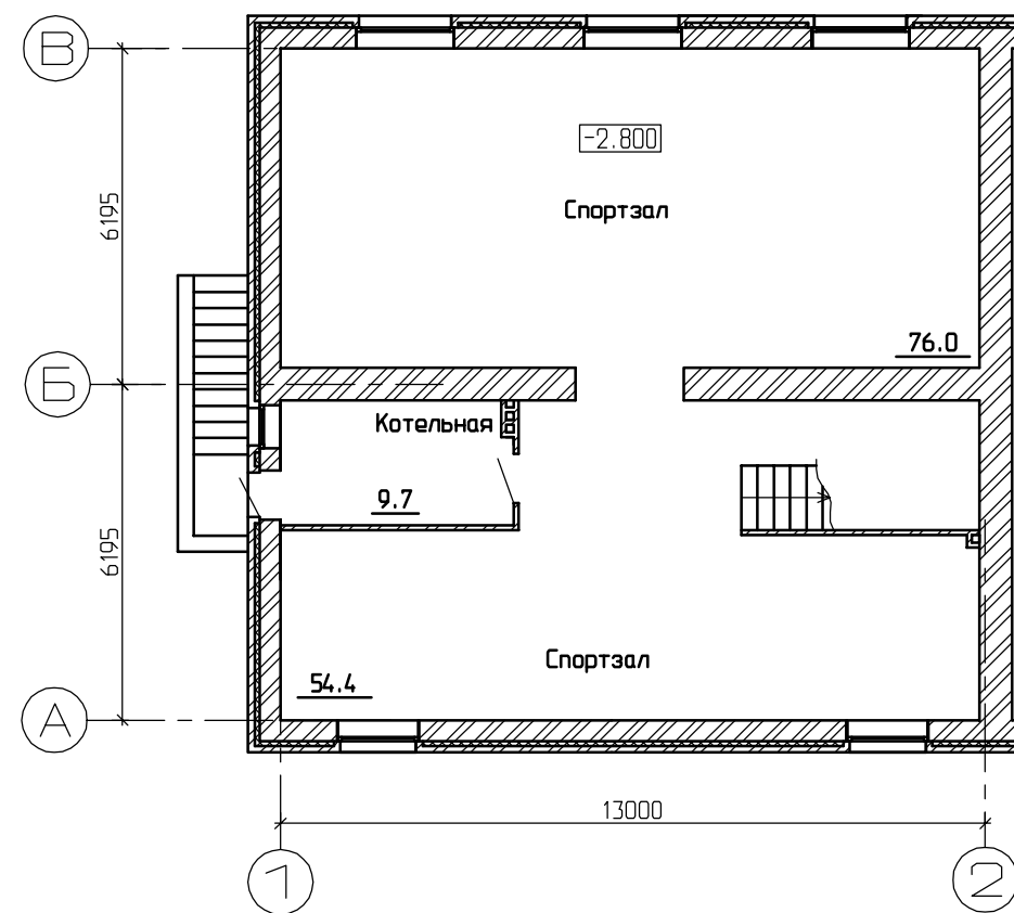
План подвала
