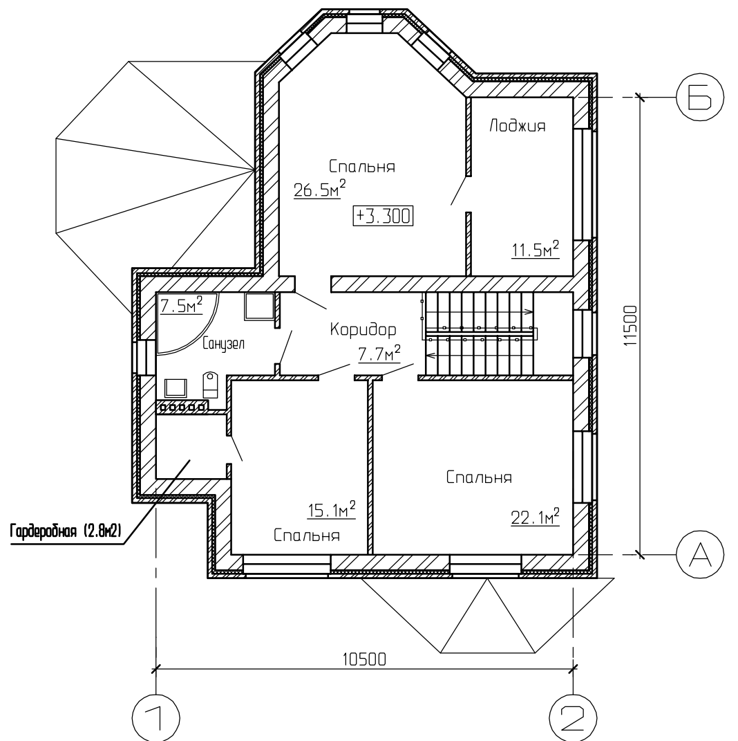
План мансарды
