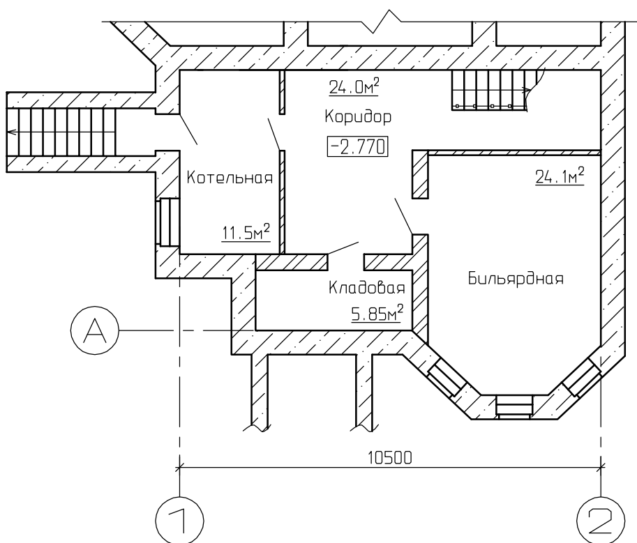
План подвала
