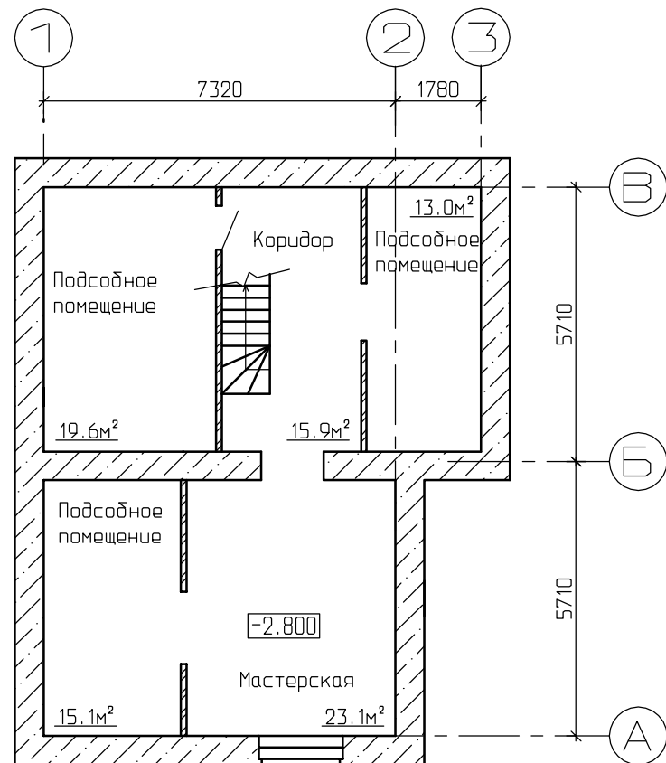
План подвала
