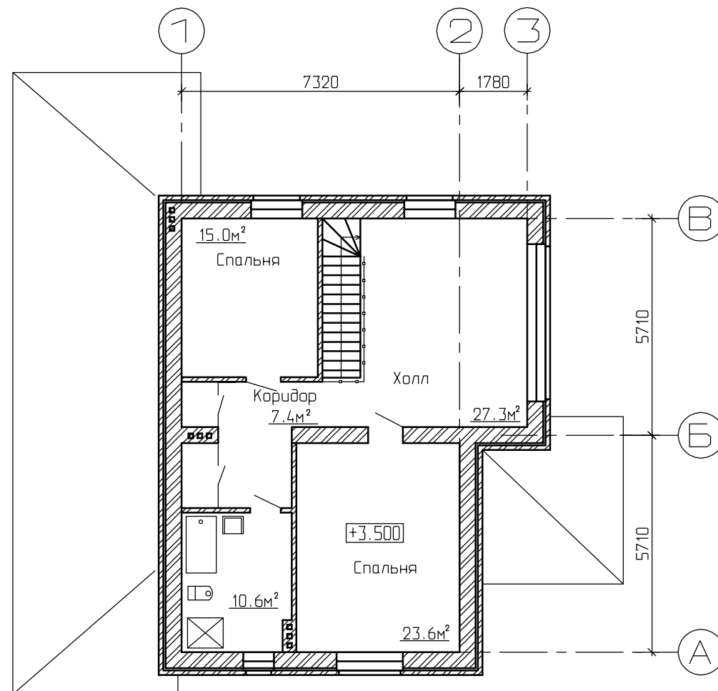
План мансарды
