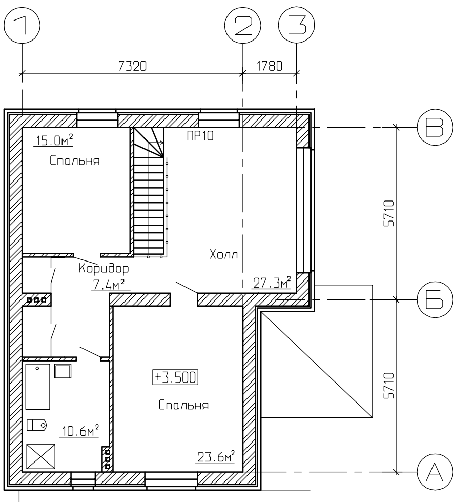
План мансарды
