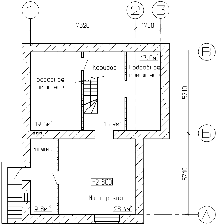
План подвала
