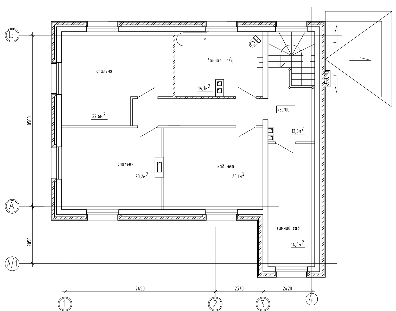
План мансардного этажа
