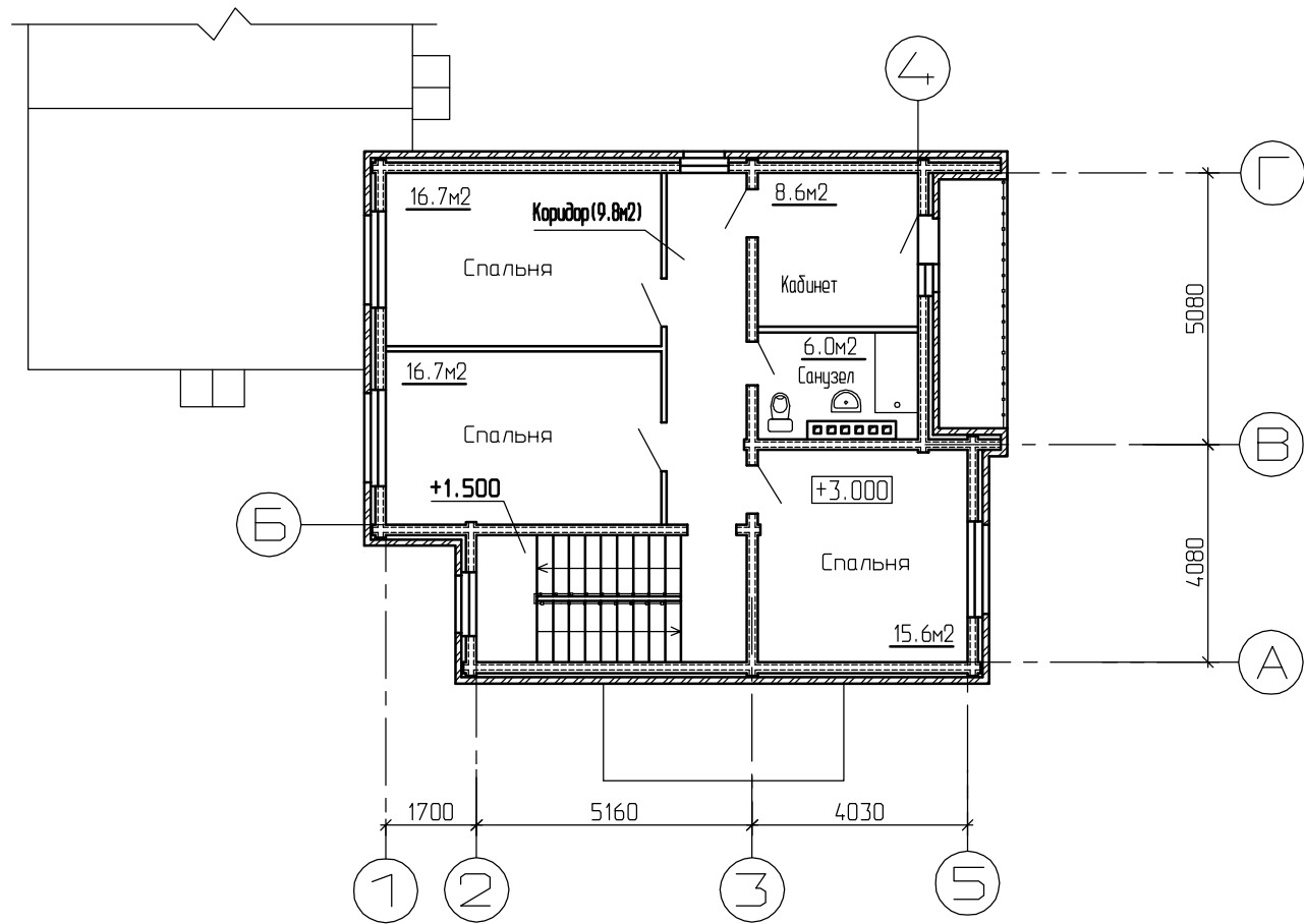
План мансарды
