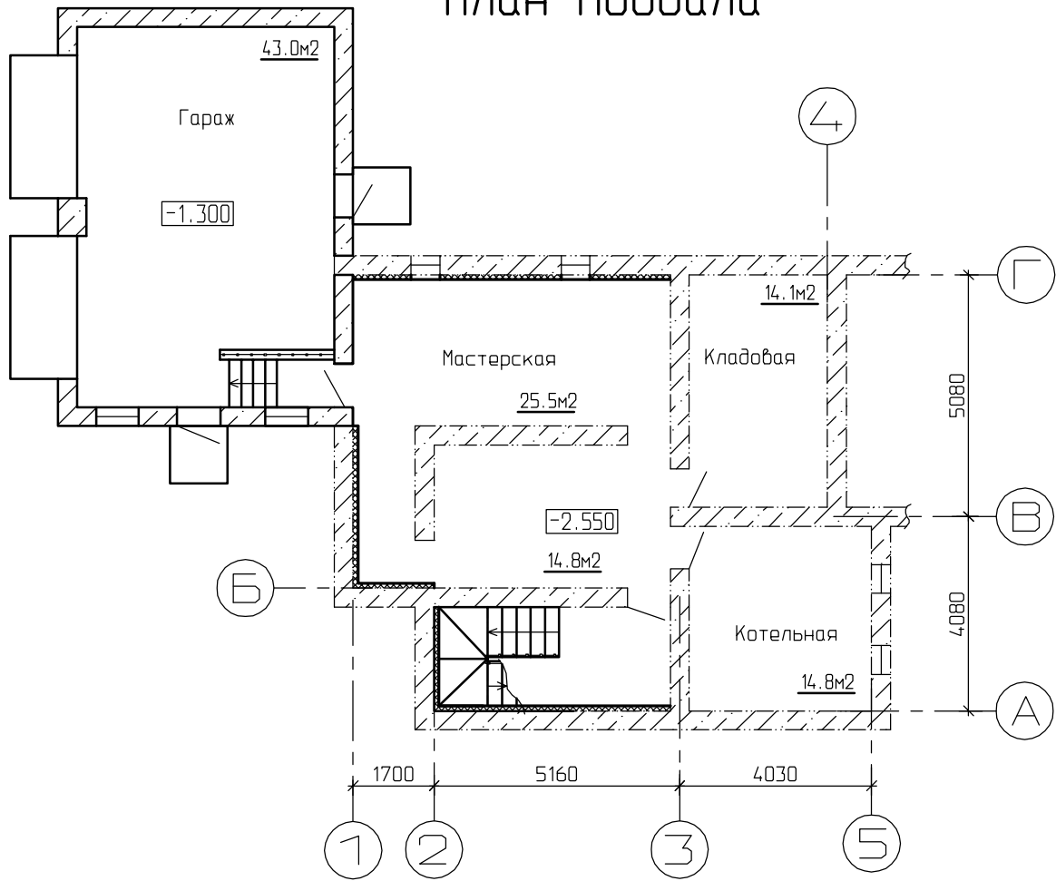
План подвала
